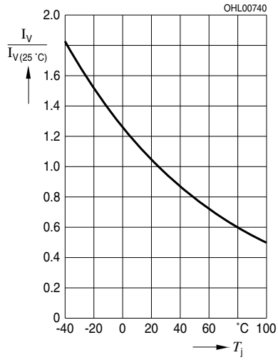
Relative Luminous Intensity 7) page 19 Relative Lichtstärke 7) Seite 19 I_V/I_V(25\text{ °C}) = f(T_j); I_F = 30\text{ mA}
