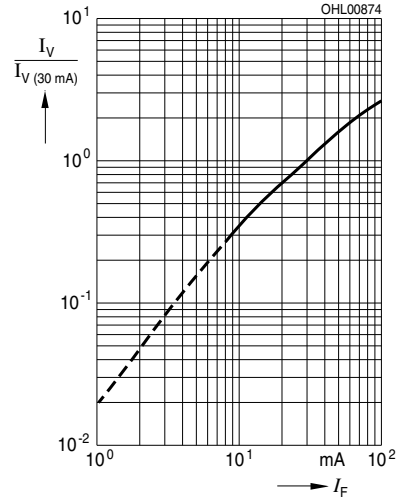
Relative Luminous Intensity 7) page 19, 8) page 19 Relative Lichtstärke 7) Seite 19, 8) Seite 19 I_V/I_V(30\text{ mA}) = f(I_F); T_S = 25\text{ °C}
