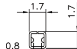
D-D SEC
