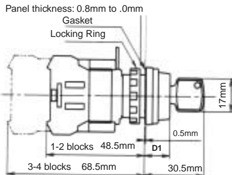
D1 = 13mm
