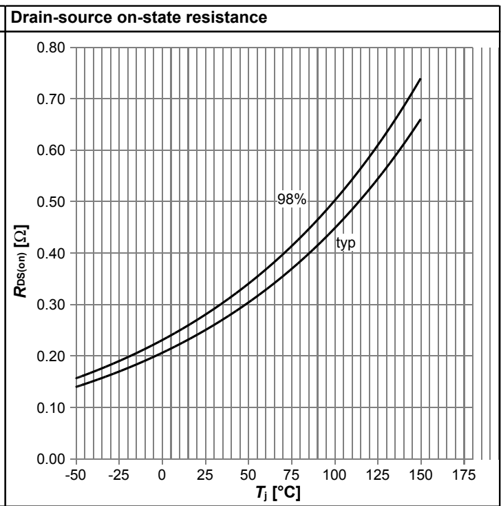
R_{DS(on)}=f(T_j); I_D=4.2\text{ A}; V_{GS}=13\text{ V}
