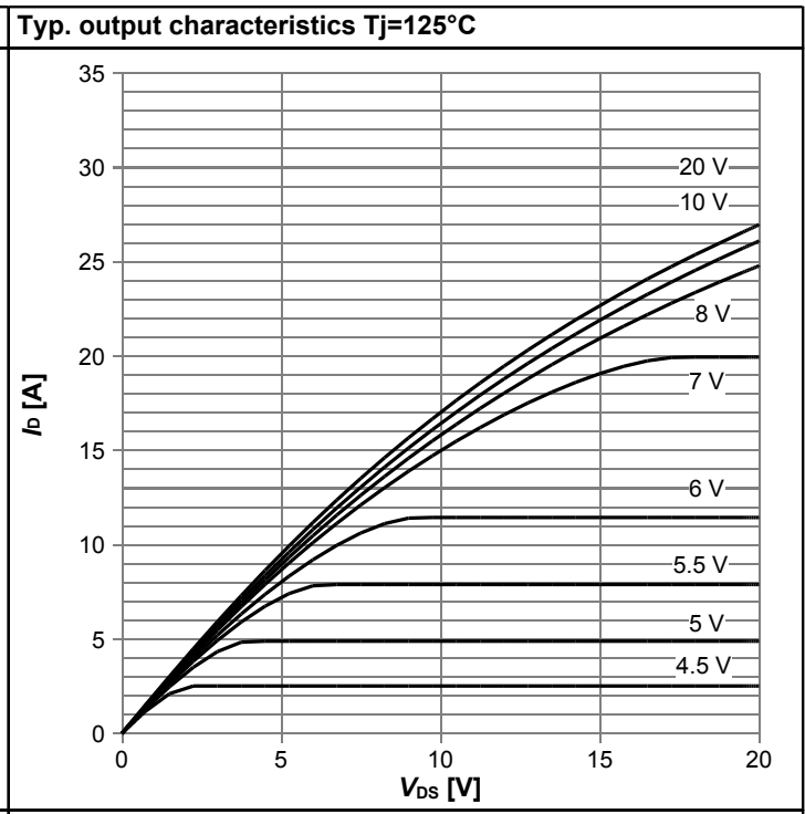
I_D=f(V_{DS}); T_j=125^\circ\text{C}; \text{parameter: } V_{GS}
