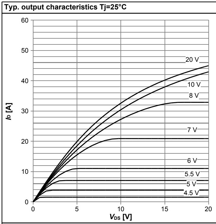
I_D=f(V_{DS}); T_j=25^\circ\text{C}; \text{parameter: } V_{GS}
