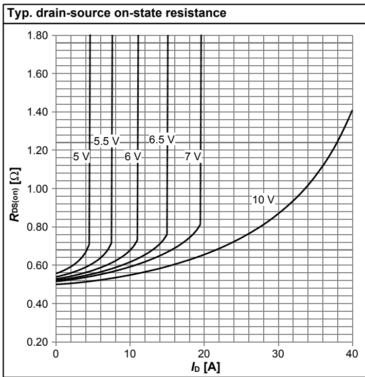
R_{DS(on)}=f(I_D); T_j=125^\circ\text{C}; \text{parameter: } V_{GS}
