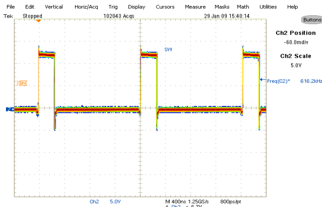
Fig. 21. Inductor node at 4A load Ch 2 : I_L
