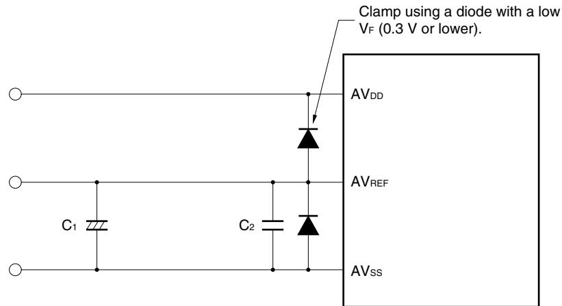
Figure 13-18. Example of Connecting Capacitor to AV REF Pin
