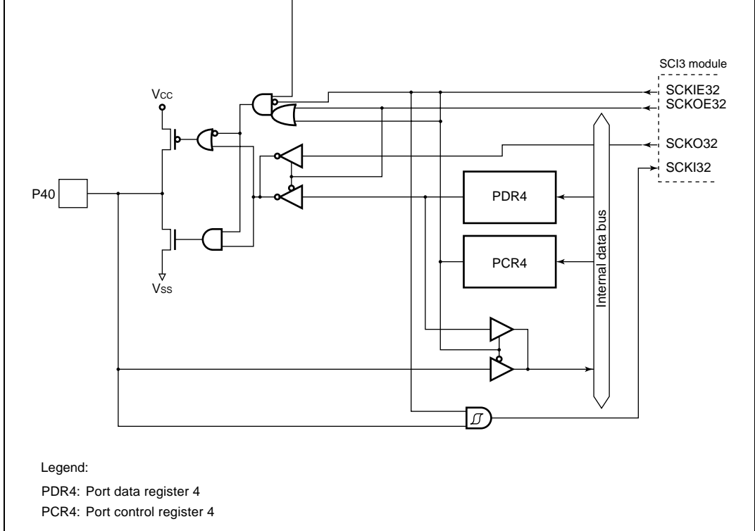
Figure B.2(d) Port 4 Block Diagram (Pin P40)
