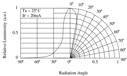
Directivity (Angle : 25^\circ )
