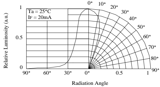
Directivity (Angle : 35^\circ )
