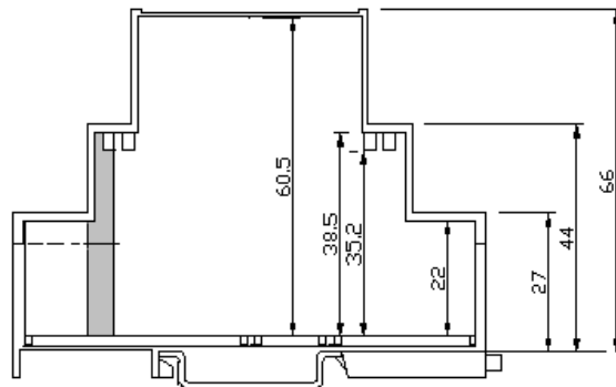
BARRA DIN
