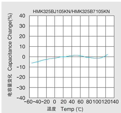
电容量—温度特性 Temperature characteristics
