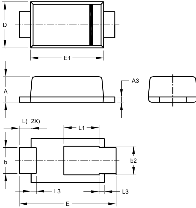
PowerDI123
