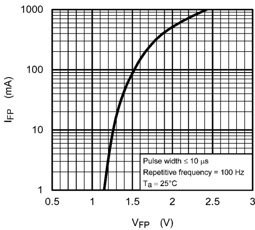
Fig. 12.5 I_{FP} - V_{FP}
