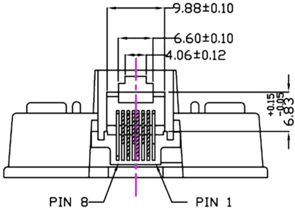
Dimensions : Millimetres
