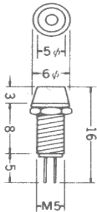
Model 407 ( 2 Volt ) 6 mm panel hole
