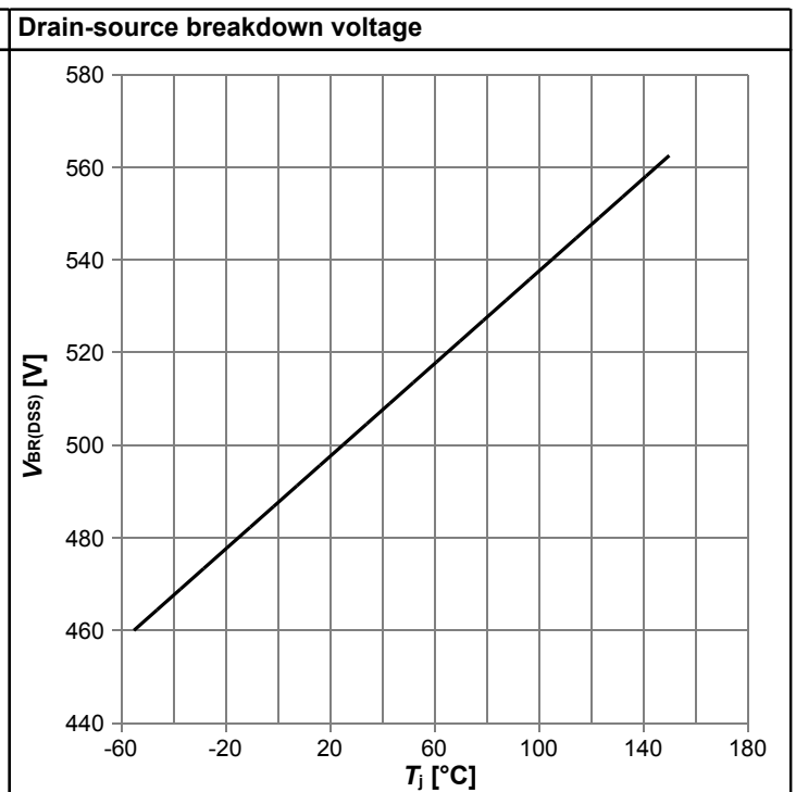
V_{BR(DSS)}=f(T_j); I_D=1 \text{ mA}
