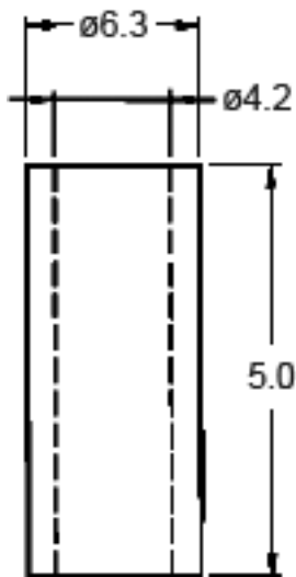
Dimensions : Millimetres
