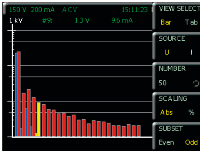
Harmonischen-Analyse: Balkendiagramm.
