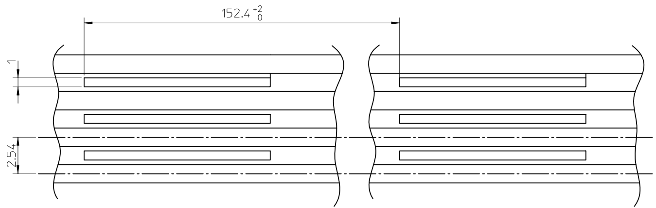
Numer narzędzia 158 - pojedyncze wycięcie Tool number 158 - single cut-out
