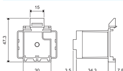
Top 35 mm rail (EN 60715) adaptor for 56.34
