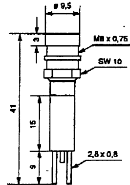
LED Signalleuchte mit Innenreflektor LED Indicator with interior reflector
