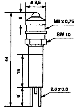
LED Signalleuchte mit Außenreflektor LED Indicator with exterior reflector
