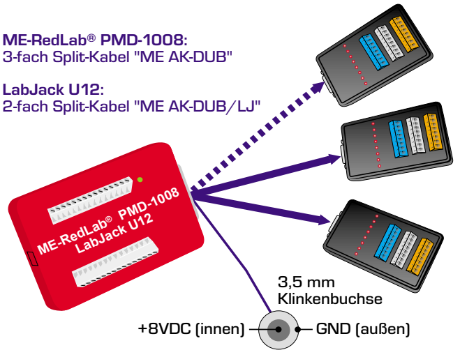
Abb. 2: Anschluß USB-Messboxen
