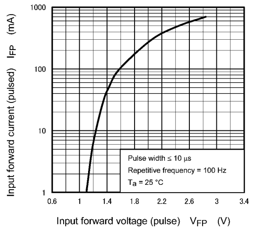
Fig. 11.6 I_{FP} - V_{FP}
