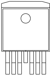
TO-263-7L
