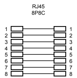
PIN Belegung / PIN wiring
