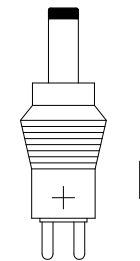
Hohlstecker/ hollowplug Ø2,5xØ5,5x12mm
