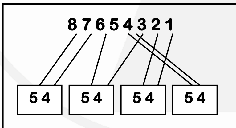
ADQ88 (Housing: Grey, Tail: Grey)
