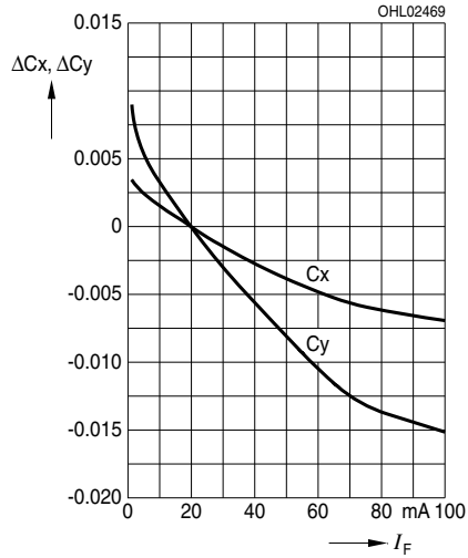
Chromaticity Coordinate Shift 6) page 23 Farbortverschiebung 6) Seite 23 C_x, C_y = f(I_F); T_S = 25\text{ °C}
