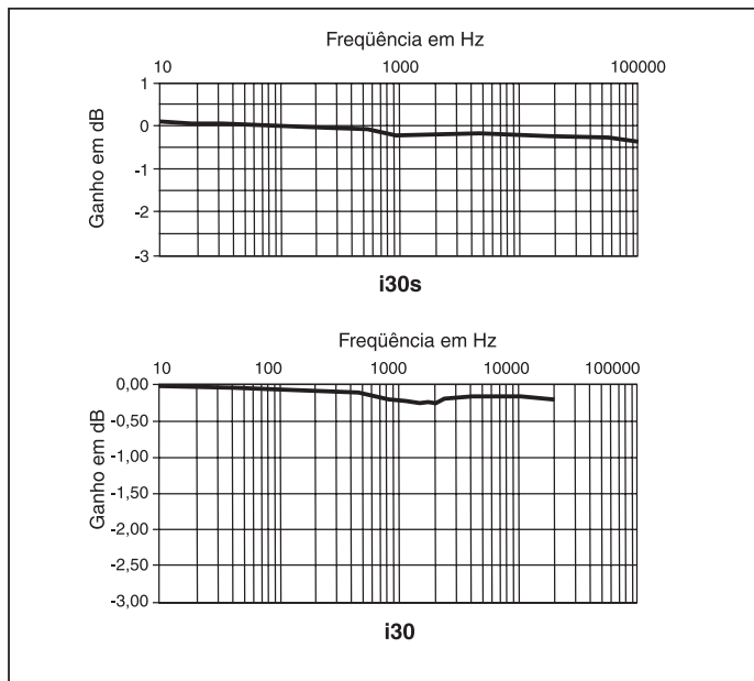
Resposta de frequência típica
