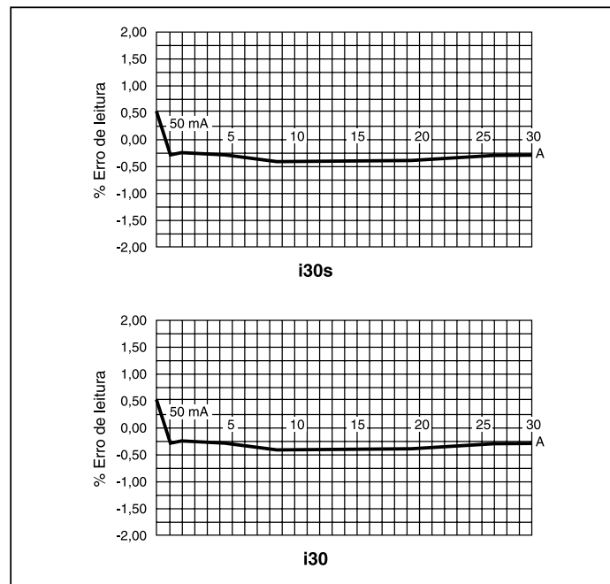
Curva de precisão típica
