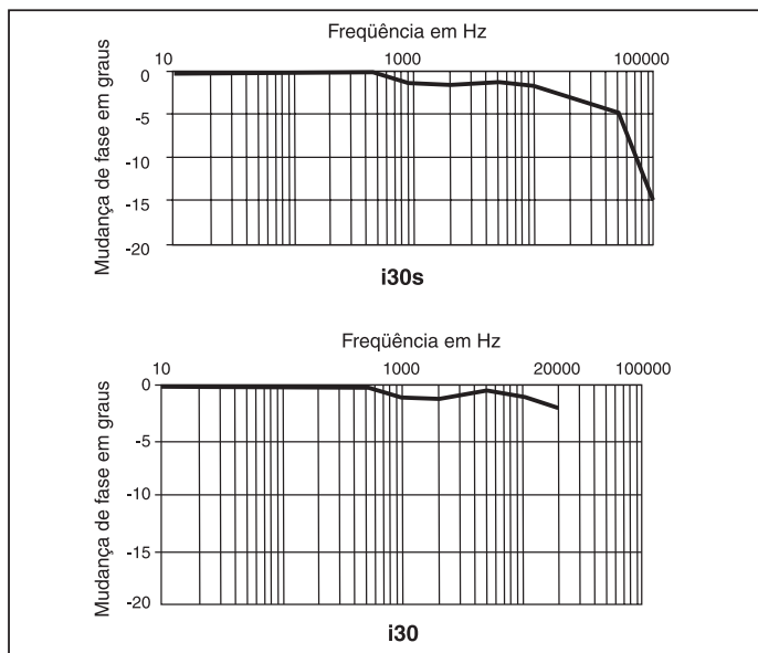
Resposta de frequência típica
