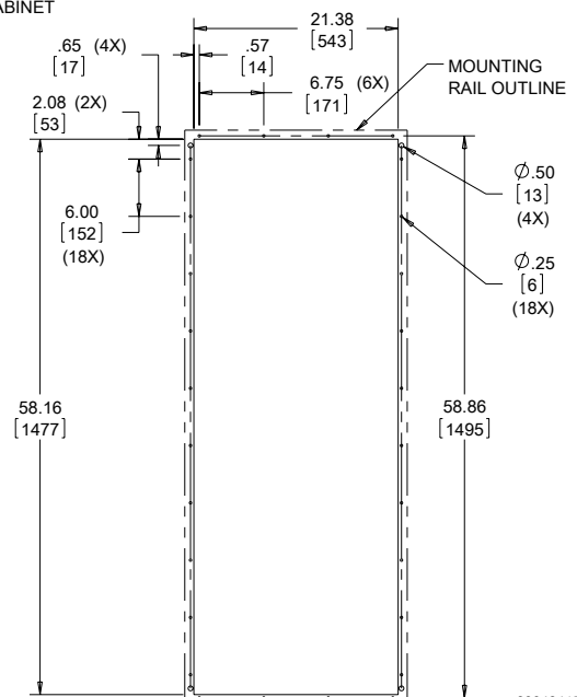
Cutout Dimensions
