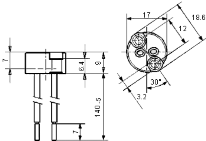
Dimensions : Millimetres
