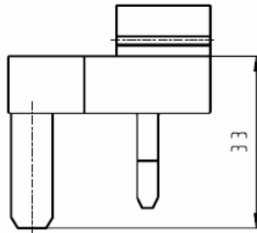
UK-Stecker/plug 1717618
