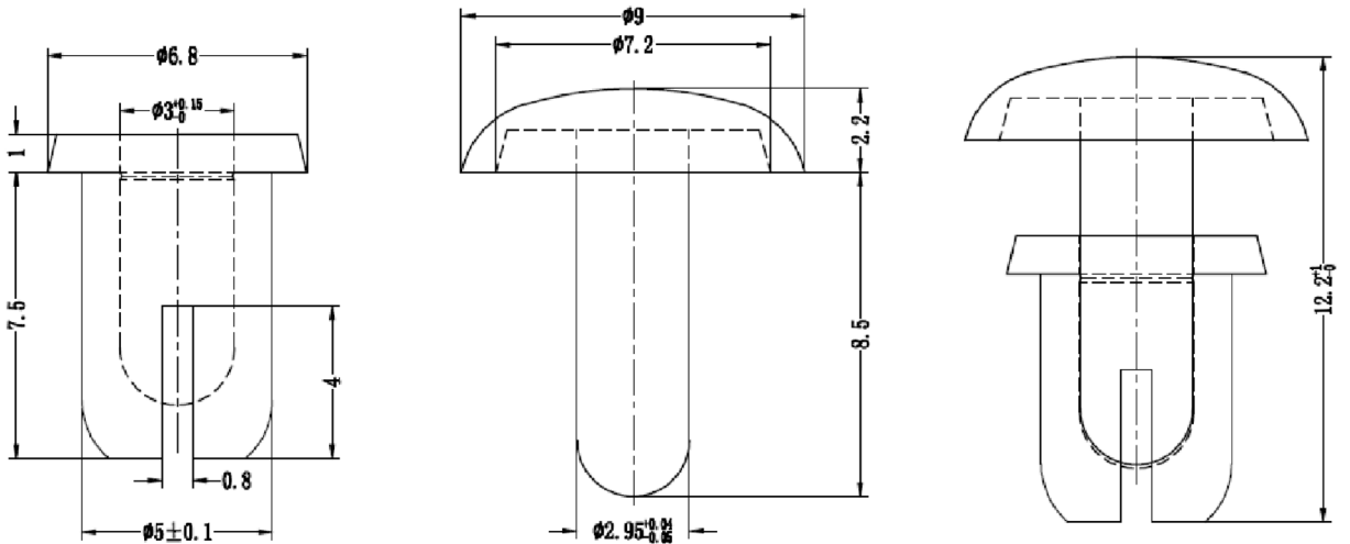
Dimensions : Millimetres
