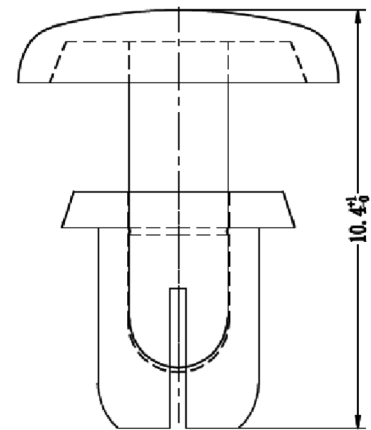
Dimensions : Millimetres
