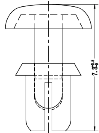
Dimensions : Millimetres
