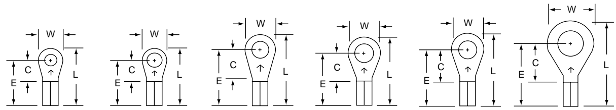
MU14-4R/S MU14-6R/S MU14-8R/L MU14-10R MU14-10R/L MU14-14R/S Stud Size 4 6 8 10 10 1/4 Wire Range 16-14 16-14 16-14 16-14 16-14 16-14
