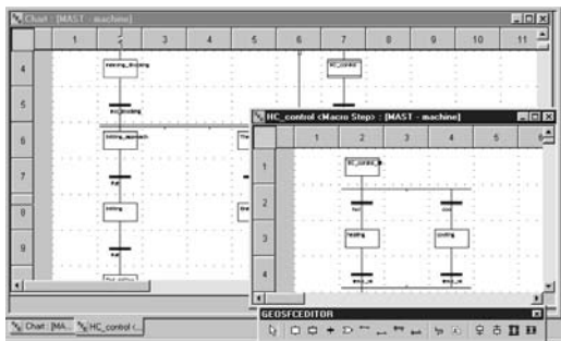
SFC charts
