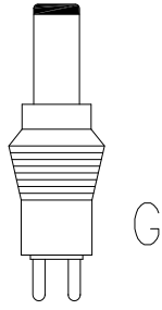
Klinkenstecker/ jackplug 3,5x15mm Art.Nr.:10950037
