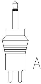
Klinkenstecker/ jackplug 2,5x12mm Art.Nr.:10950038
