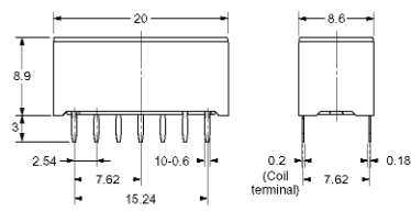
G6ZK-1P
