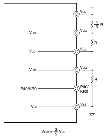
(d) 1/2 bias method (MDSET1, MDSET0 = 0, 0) (example of V_{DD} = 5\text{ V} , V_{LC0} = 3\text{ V} )
