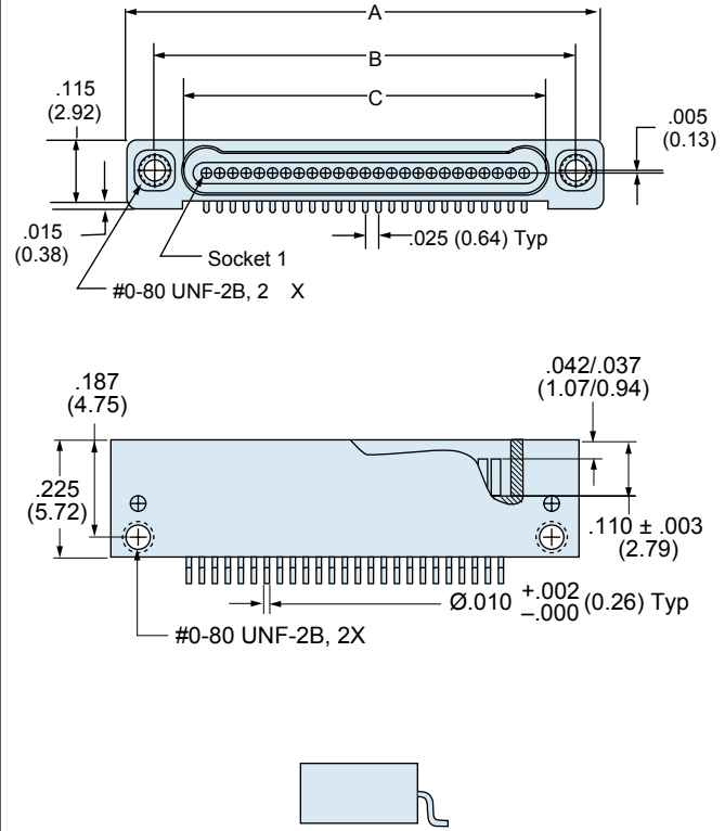
890-013 Receptacle (Socket) Connectors
