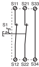
Fig. 3: Solo PNOZ X2.1: rearme automático/Solo PNOZ X2.1: Start automat./Alleen bij PNOZ X2.1: automat. start
