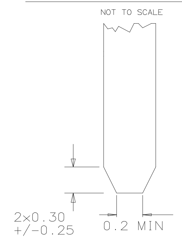
CARD EDGE CONNECTOR BEVEL
