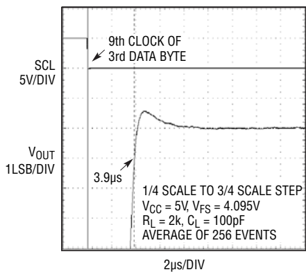
2 \mu\text{s} /DIV
