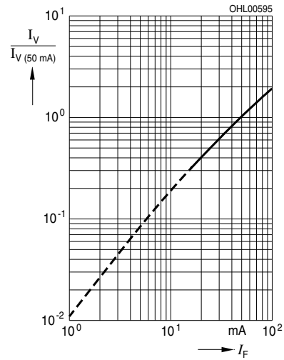
Relative Luminous Intensity 7) page 19, 8) page 19 Relative Lichtstärke 7) Seite 19, 8) Seite 19 I_V/I_V(50\text{ mA}) = f(I_F); T_S = 25\text{ °C}
