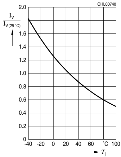
Relative Luminous Intensity 7) page 19 Relative Lichtstärke 7) Seite 19 I_V/I_V(25\text{ °C}) = f(T_j); I_F = 50\text{ mA}
