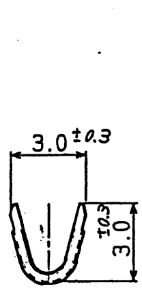
A-A SEC.
