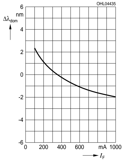
Dominante Wellenlänge 2) Seite 23 Dominant Wavelength 2) page 23
