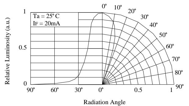
Directivity (Angle : 35°)
