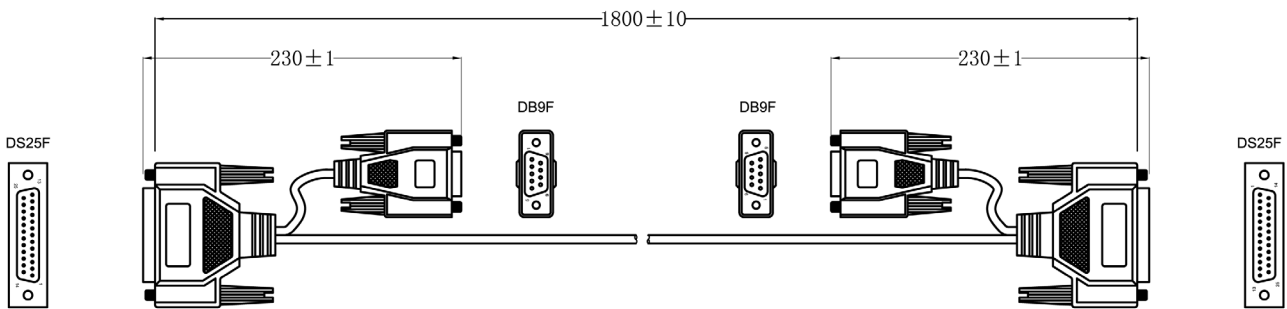
Dimensions : Millimetres
