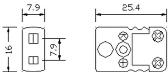
Miniature Socket
