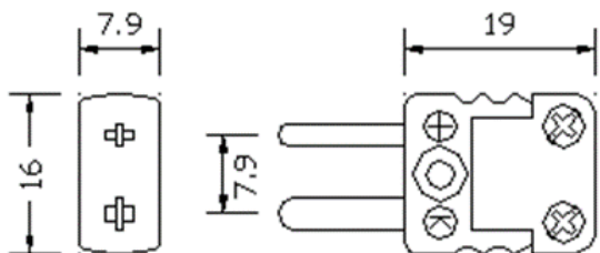
Miniature Plug
